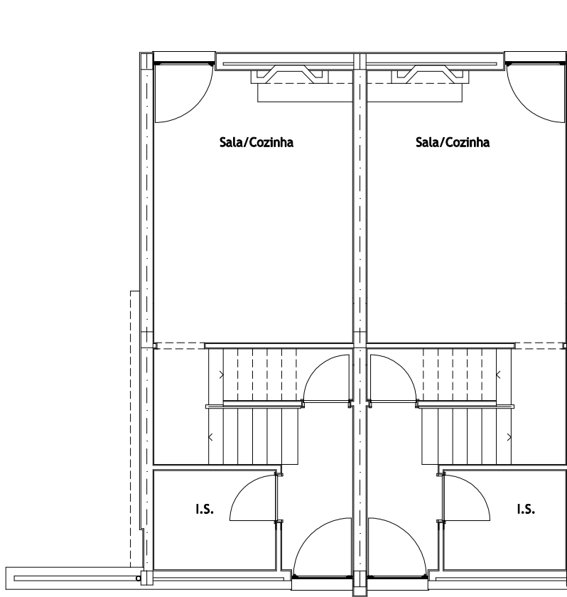
PLANTA DO PISO 0
